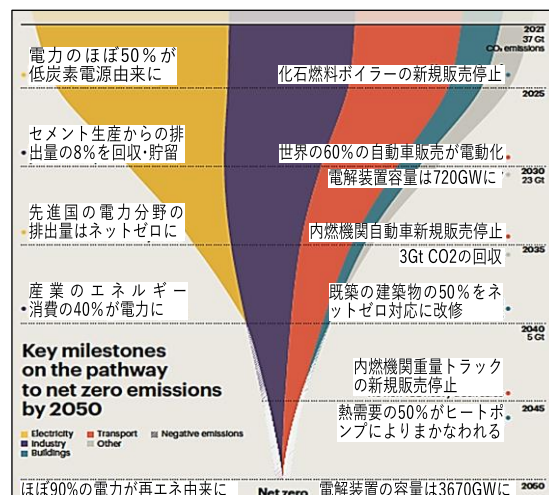
図2 2050年ネットゼロへの道筋 出典：IEA, 2022
