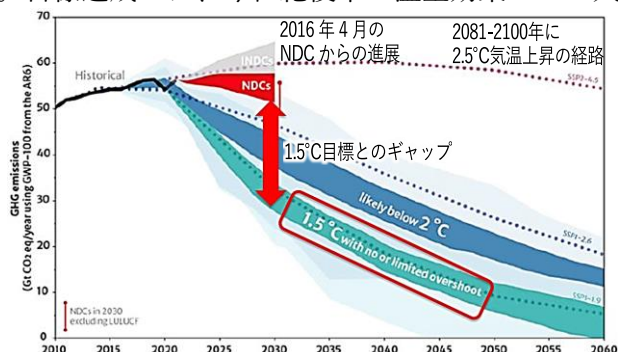
図1 1.5℃目標と削減目標(NDC)(2022/9)のギャップ
